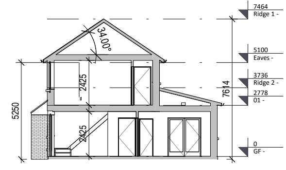
6 Section B-B 1 : 200
